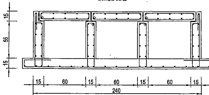
CANIVEAU TRIPLE
