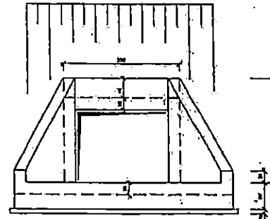
ELEVATION AMONT vue 1/20
