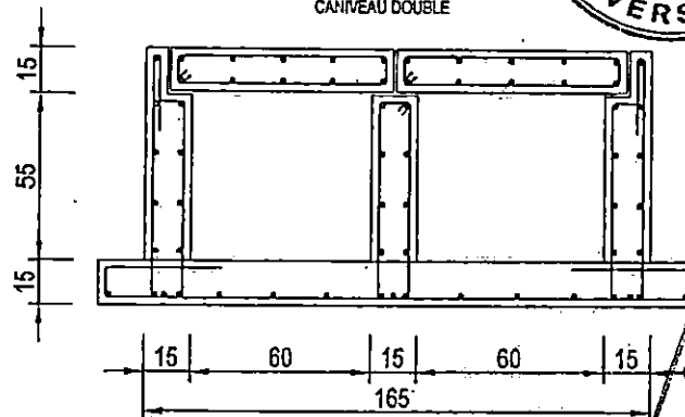
CANIVEAU DOUBLE
