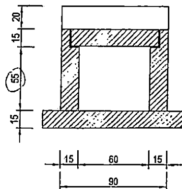
COUPE TRANSVERSALE
