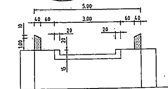
COUPE A-A
